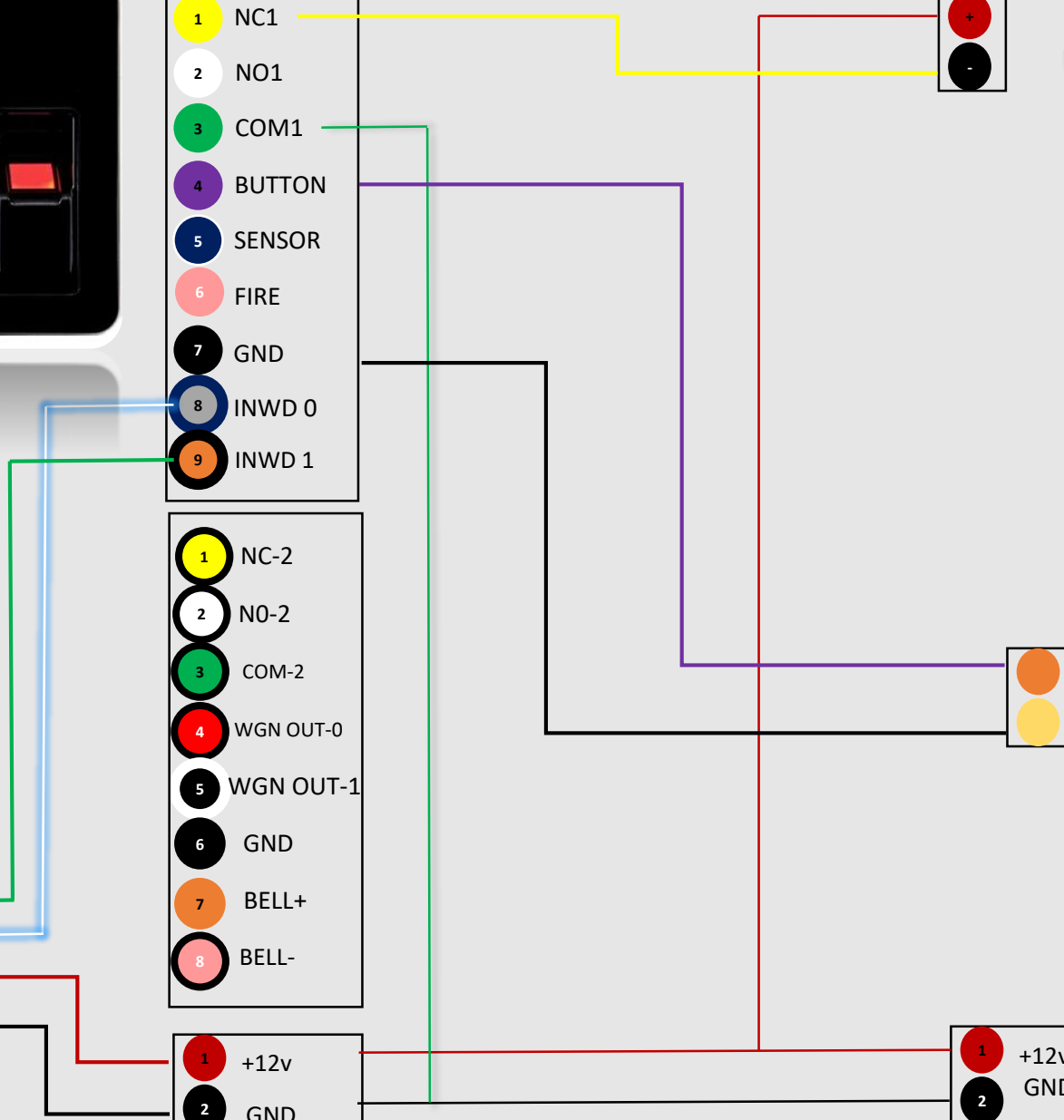
EM Lock
